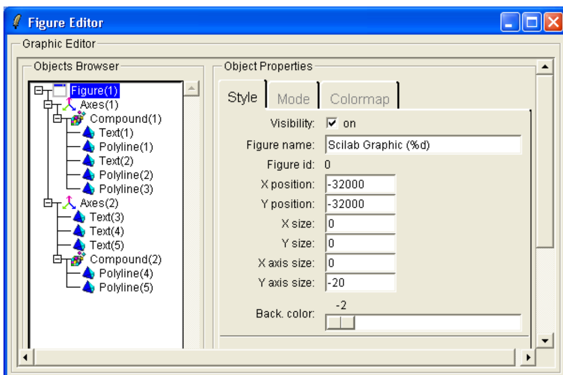
Figura 4.12. Editor de gráfico associado à figura 4.5
