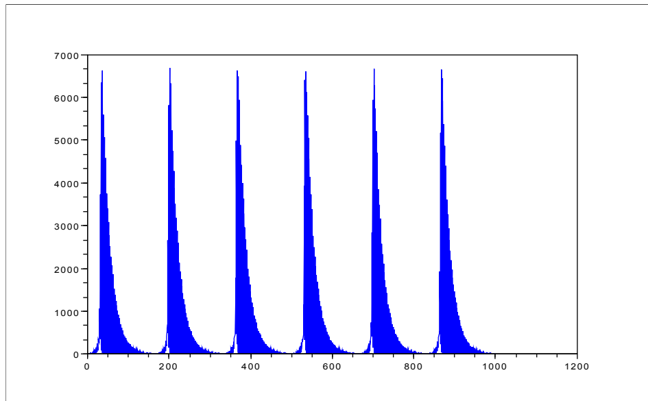
Figura 5.8. Gráfico da solução do sistema de duas EDO, criado pelo comando plot(ode(y0,t0,t,f))
