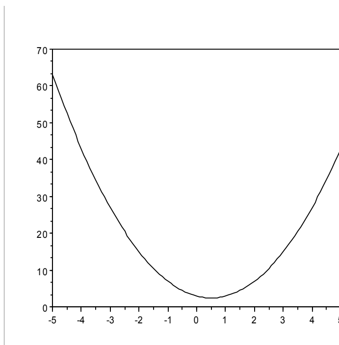
Figura 5.11. Gráfico da função minimizada
