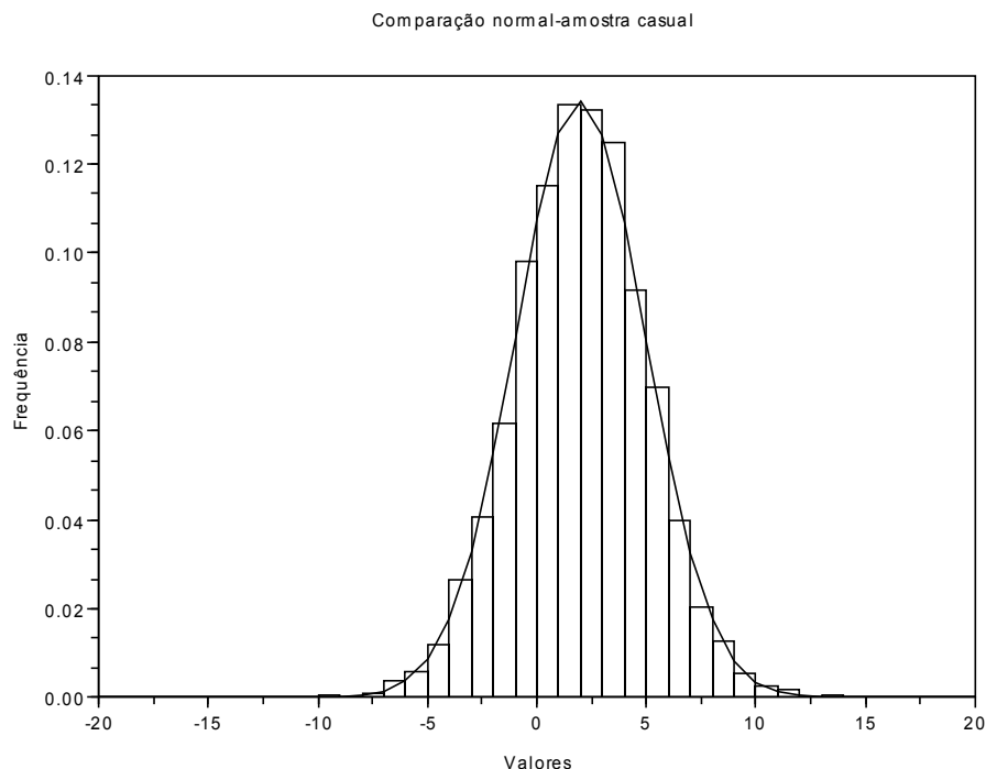
Figura 2.13. Comparação entre o histograma de uma amostra de distribuição normal e a curva normal associada
