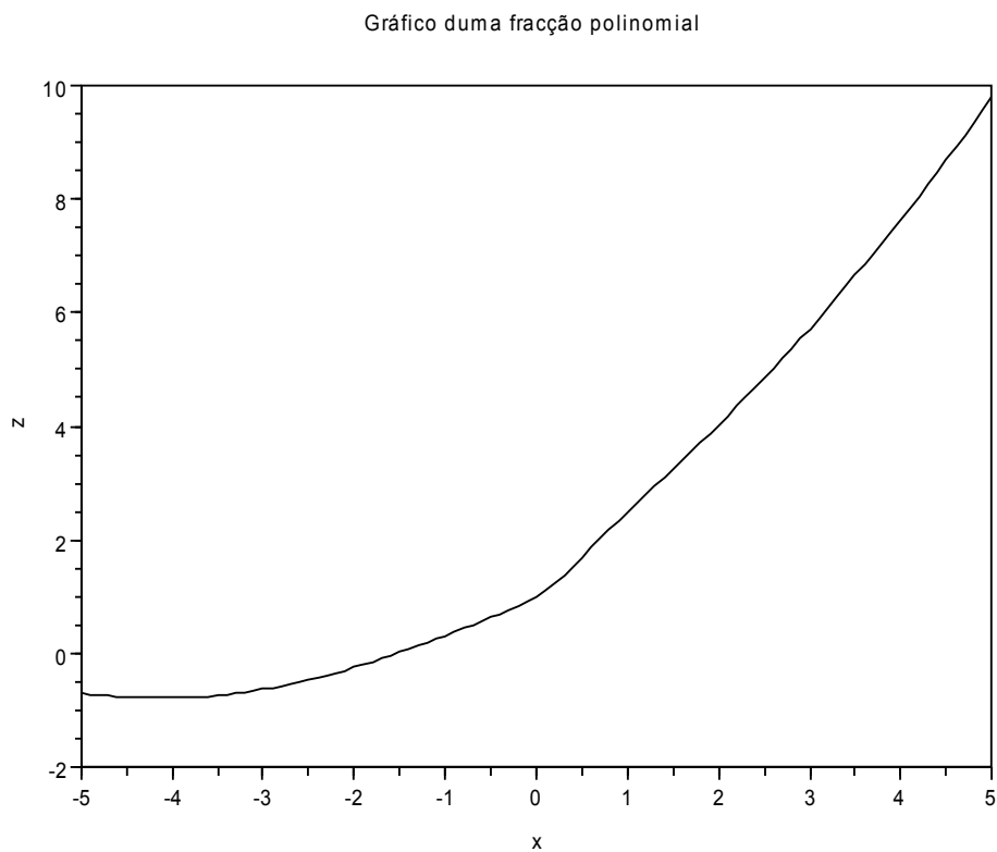
Figura 2.10. Gráfico da fracção polinomial z
