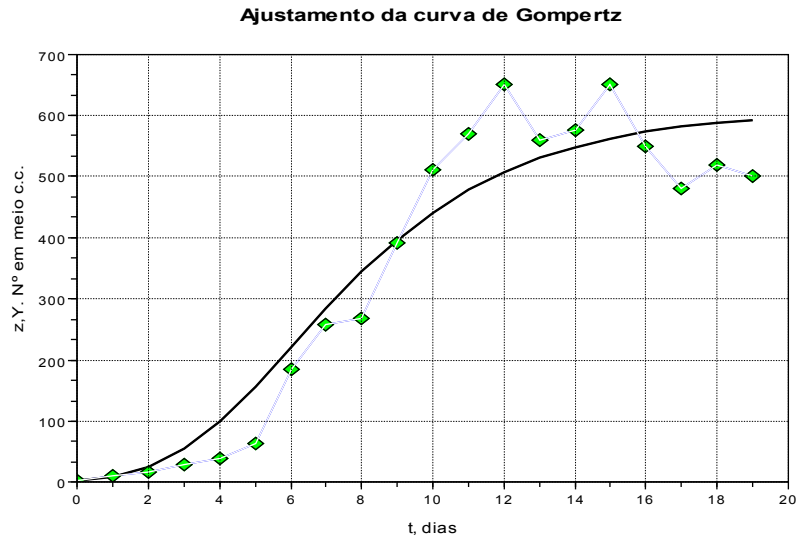
Figura 5.1. Aplicação do comando datafit. Valores medidos e simulados pelo ajustamento de uma curva de Gompertz a dados de Gause, de uma cultura pura de Paramecium aurelia
