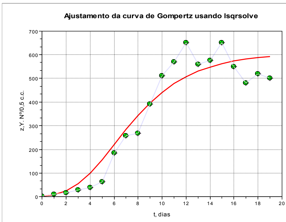
Figura 5.2. Aplicação do comando lsqrsolve. Valores medidos e simulados pelo ajustamento de uma curva de Gompertz a dados de Gause, de uma cultura pura de Paramecium aurelia
