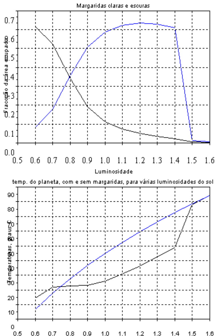
Figura 8.14. Dinâmica do planeta das margaridas associada à variação da luminosidade da sua estrela.. Gráfico superior: variação das frações das duas áreas (cor preta associada à margarida escura). No gráfico inferior, a estrela do planeta é designada abreviadamente por sol, e a linha a azul corresponde ao planeta sem vegetação
