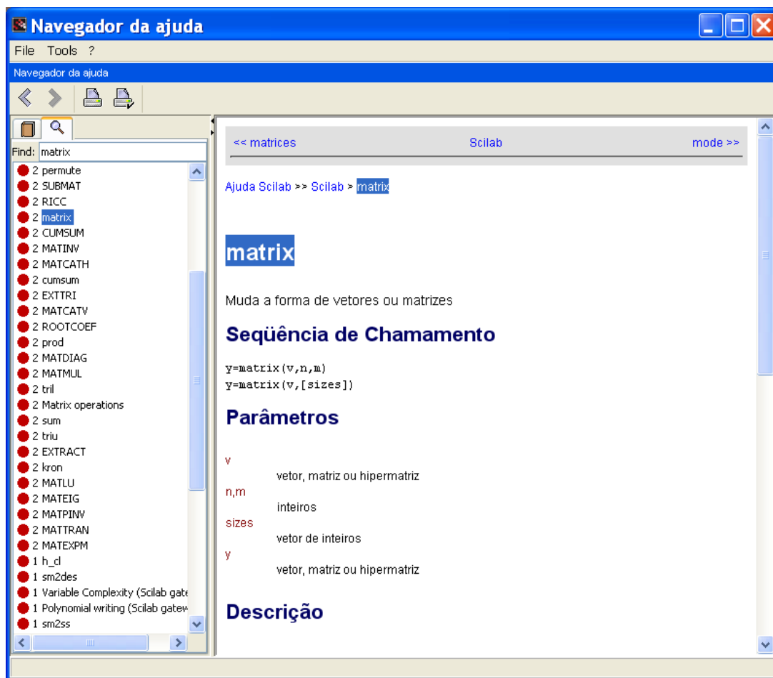
Figura 1.4. Janela da ajuda que surge depois de se ter: a) pressionado a tecla F1; b) no local para a palavra a ser procurada (Find) termos escrito “matrix”; c) de entre as varias alternativas apresentadas termos escolhido “matrix”
