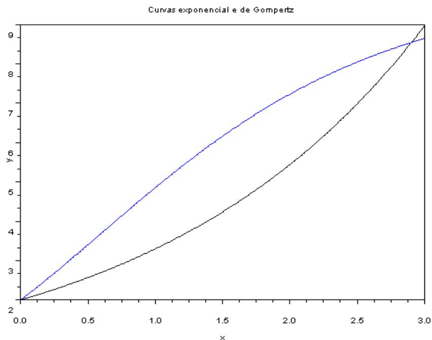
Figura 2.3. Gráfico de uma curva exponencial e outra de Gompertz
