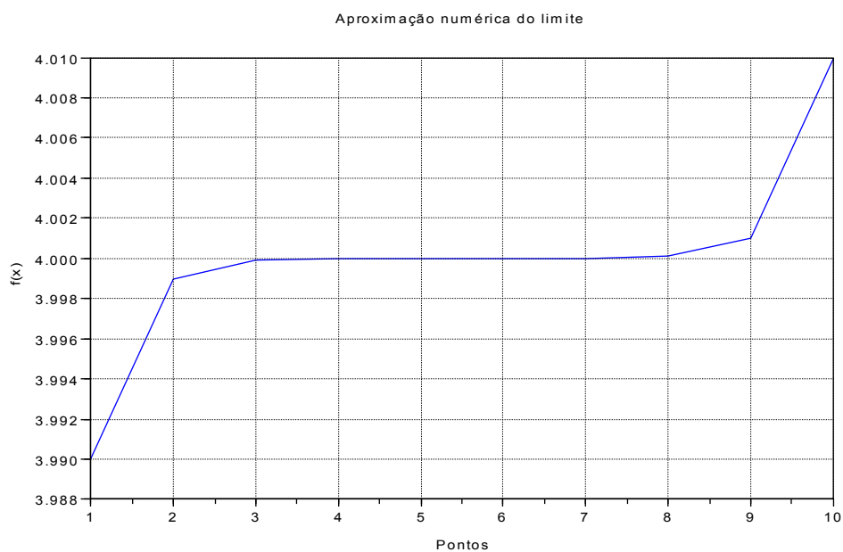
Figura 2.11. Aproximação numérica do limite da função f(x)=(x^2-4)/(x-2)
