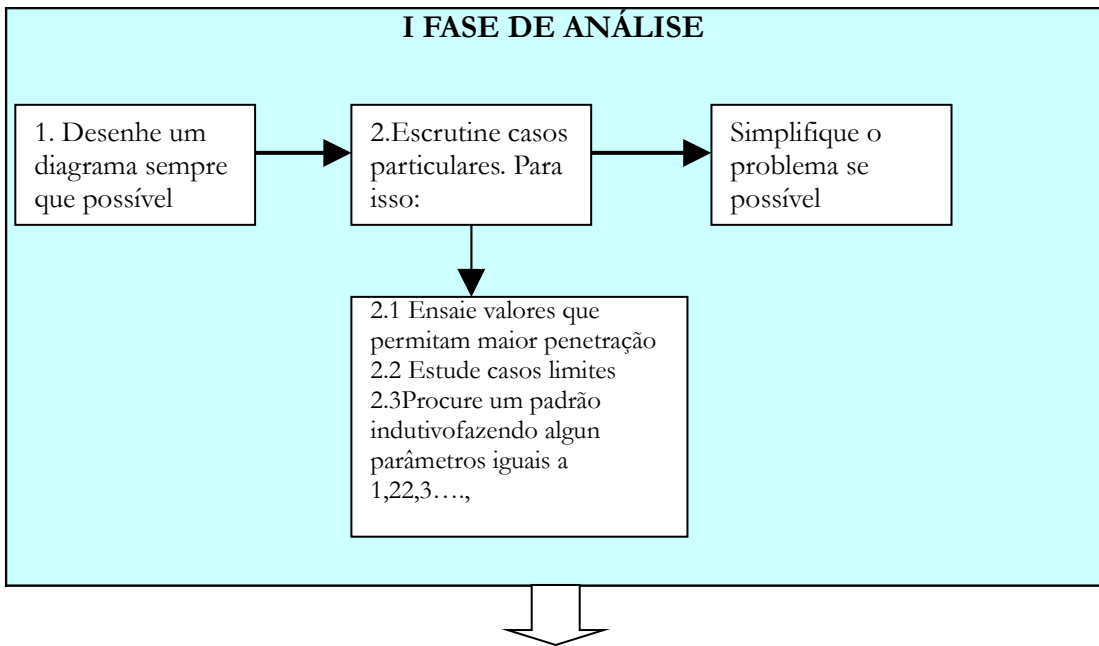
Figura 6.2. Diagrama da heurística de A. H. Schoenfeld
