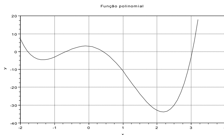
Figura 2.7. Gráfico da função polinomial definida
