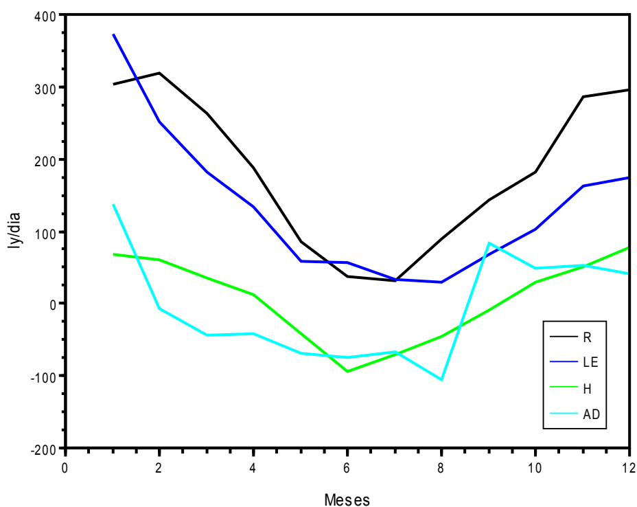
Figura 8.11. Estimativa preliminar do balanço da energia na região de Maputo. R - balanço da radiação; LE – energia consumida na evapotranspiração; H – fluxo de entalpia solo-atmosfera; AD – aquecimento ou arrefecimento do solo, mais advecção ou dissipação de energia. A unidade utilizada é o ly/dia. (Barreto, 1974)
