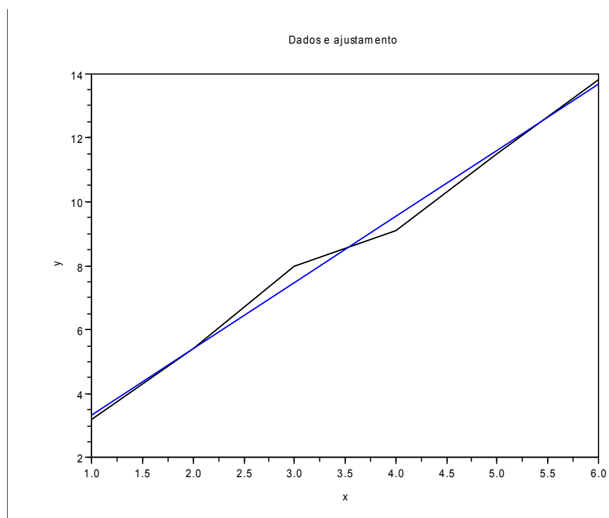
Figura 3.1. Dados e reta ajustada
