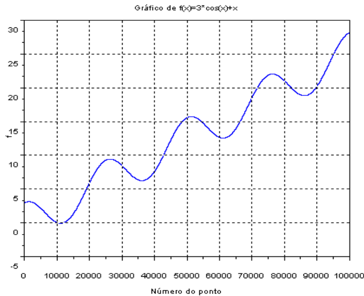
Figura 2.5. Gráfico da função trigonométrica f(x)=3 \cos x + x
