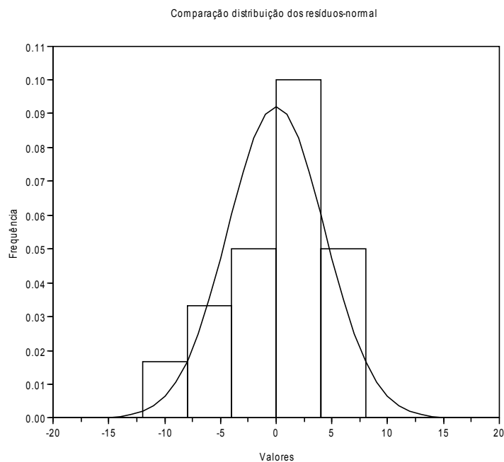
Figura 8.2. Segunda saída de gráficos do programa reglinmul. Comparação da distribuição dos resíduos com a distribuição normal
