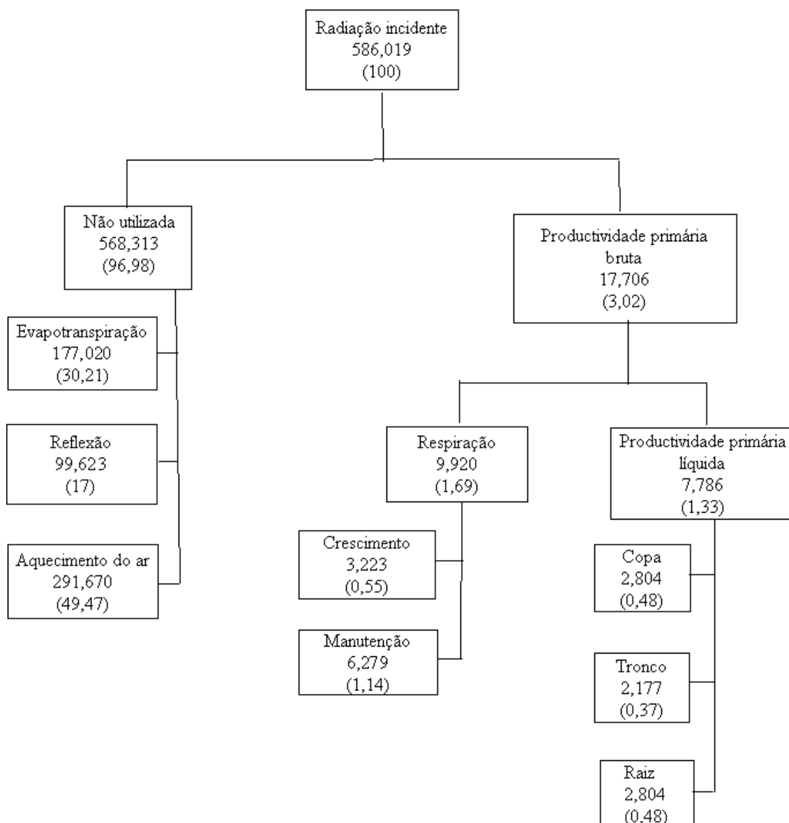
Figura 8.12. Pinhal bravo regular aos trinta anos, numa estação de boa qualidade. Primeira estimativa do balanço da radiação. Valores referidos a 10^8 \text{ kJ ha}^{-1} \text{ ano}^{-1} . Os valores entre parêntesis são a correspondente percentagem referida à radiação solar incidente. Barreto (2000, 2004a)
