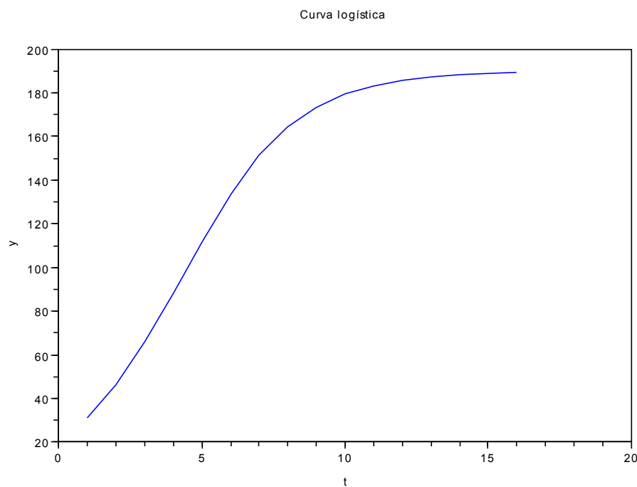
Figura 5.9. Solução da equação de diferenças da curva logística
